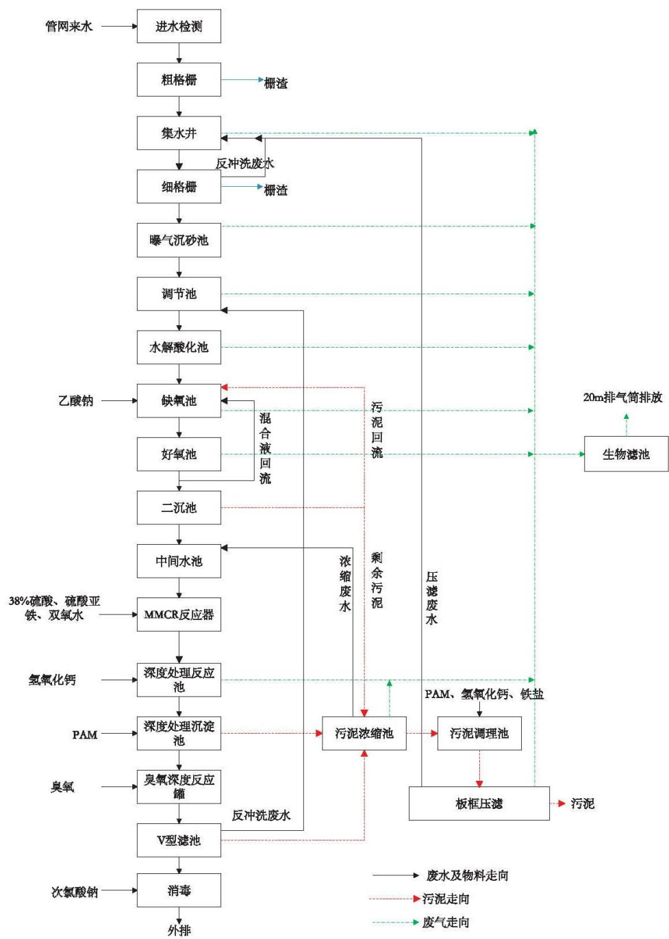
图 5.4-1 园区污水处理厂处理工艺流程图
