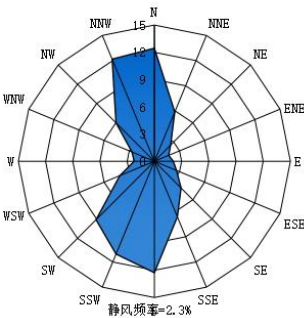
图 4.4-1 文登近 20 年（2005～2024 年）风向频率玫瑰图
